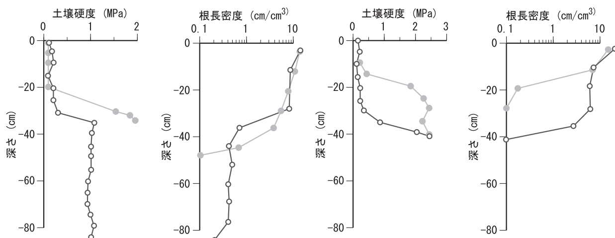
図4 土層内における貫入式土壌硬度計による土壌硬度および小麦の根長密度の分布（北見農試 2002）
