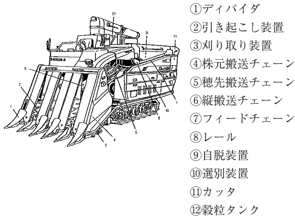
図Ⅷ-27 自脱コンバインの構造
