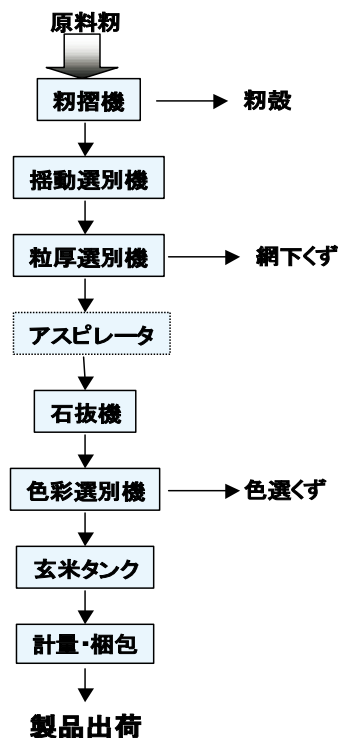
図Ⅷ－48 粳摺り、選別、調製ライン
