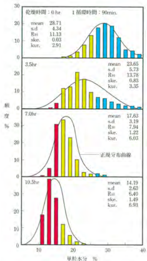
図Ⅷ－33 乾燥中の粉単粒の水分分布（笠原ら）
