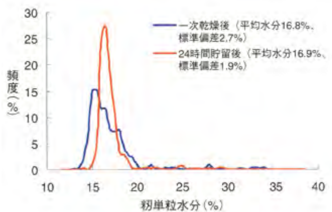
図Ⅷ-35 貯留時の単粒水分分布の変化 (中央農試)
