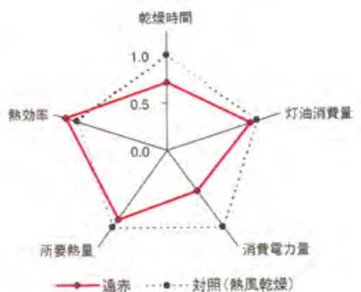
図Ⅷ-41 遠赤外線乾燥の省エネ効果
