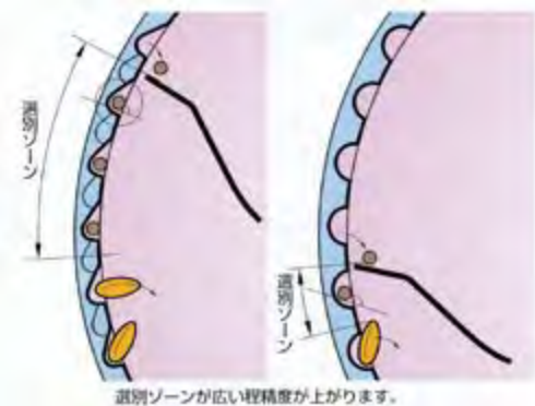
図Ⅷ－47 インデントシリンダセパレータ（HYDE社）
