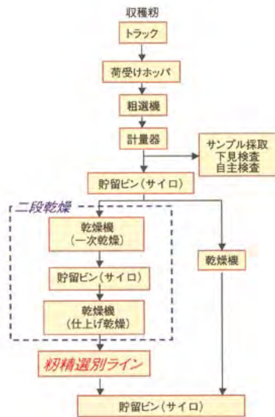
図Ⅷ－45 共同乾燥調製貯蔵施設における荷受けから乾燥終了までの選別調製ライン
