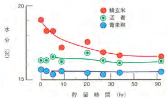
図Ⅷ-37 二段乾燥後の水分変化 (山形農試)
