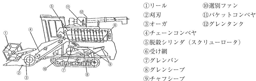
図Ⅷ－29 汎用コンバインの構造
