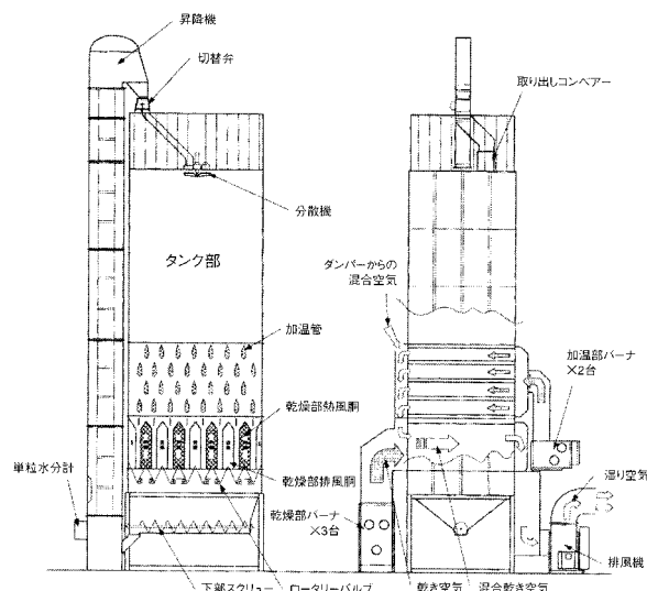
図Ⅷ－44 加温管方式の乾燥機
