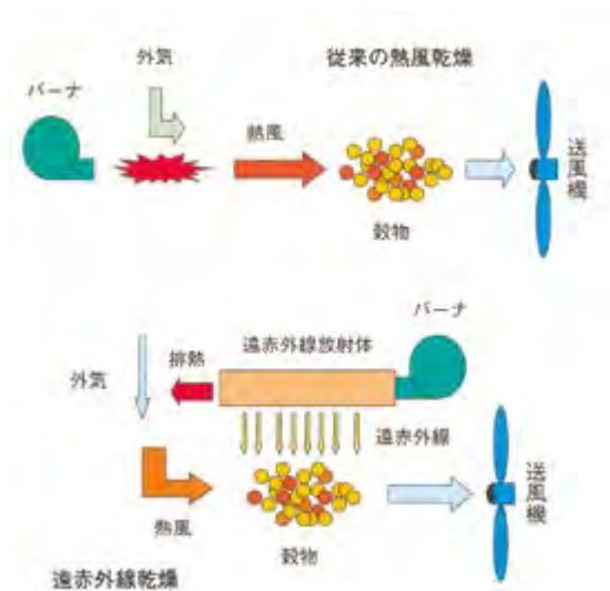
図Ⅷ-39 遠赤外線乾燥の模式図
