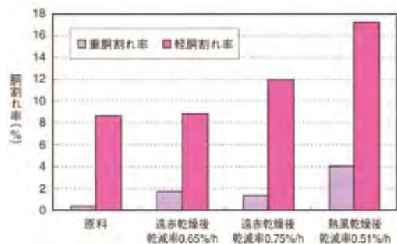
図Ⅷ-42 乾燥条件と胴割れ率
