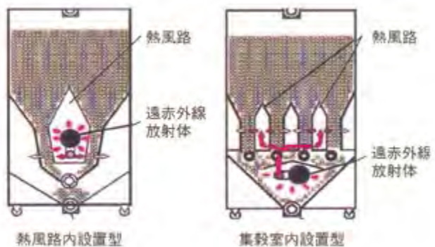
図Ⅷ-40 遠赤外線乾燥の種類
