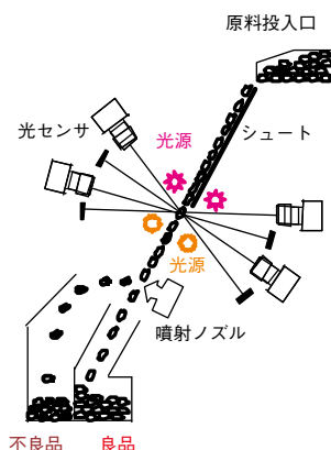
図Ⅷ－50 色彩選別機の選別方法
