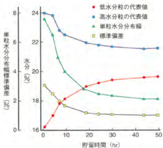
図Ⅷ-34 貯留中の粒間水分移動
