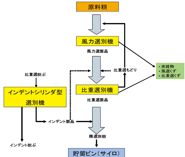
図Ⅷ－46 共同乾燥調製・貯蔵施設における貯蔵前の粳の精選別調製ライン
