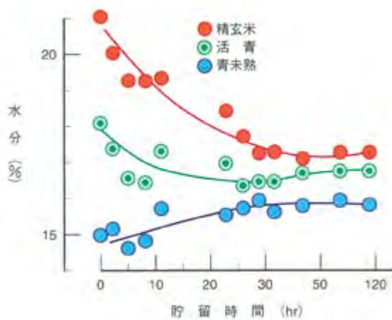
図Ⅷ-36 一次乾燥後の水分変化 (山形農試)
