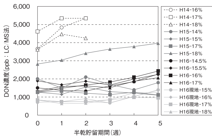
図9 半乾貯留中のDON濃度の推移
