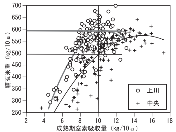
図20 成熟期窒素吸収量と精玄米重の関係
