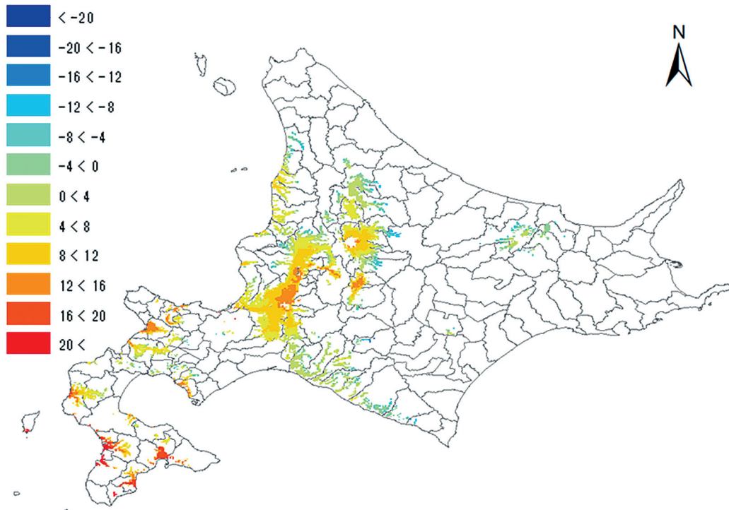
図24 密短苗「えみまる」の出穂期晩限～推定出穂期の日差マップ
