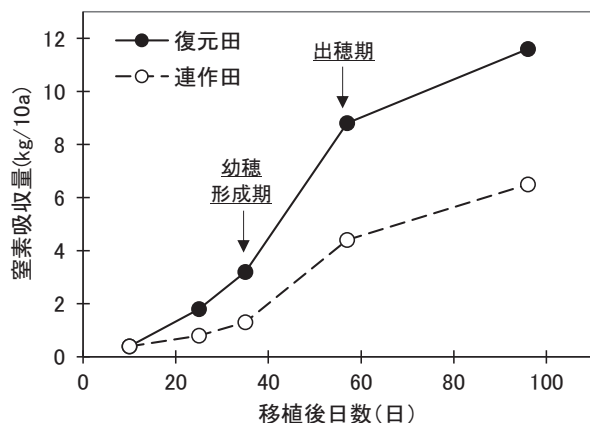
図27 復元田における水稻の窒素吸収量(北村1984)
