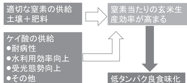
図13 良食味米生産におけるケイ酸の役割
