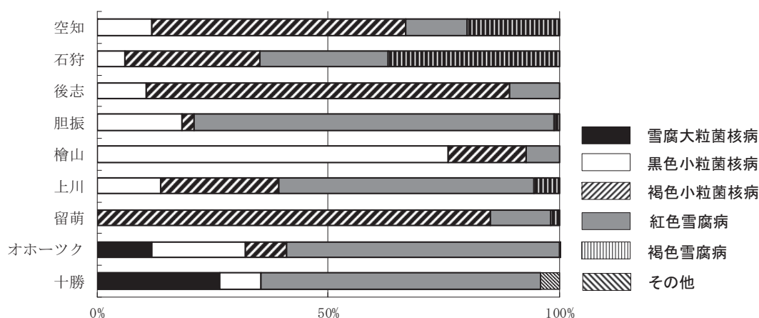
図3 小麦雪腐病の振興局別菌種別割合 (2023年4月)
