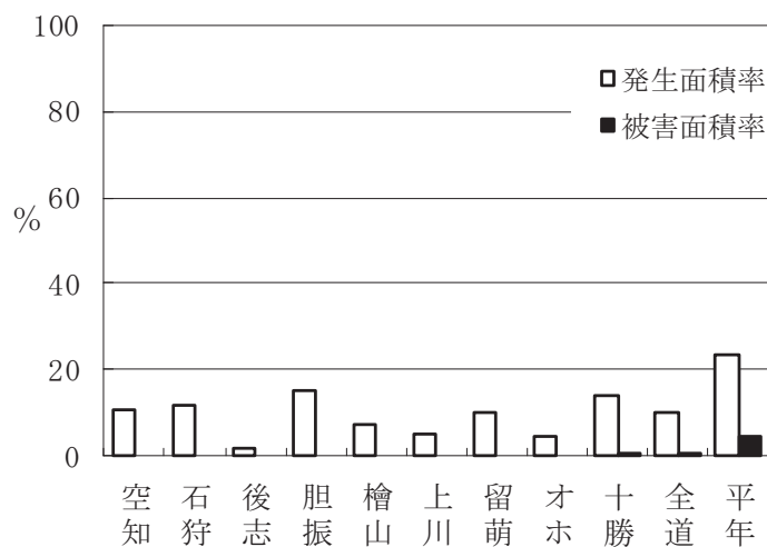
図7 振興局別の秋まき小麦赤かび病発生状況（2023年）
