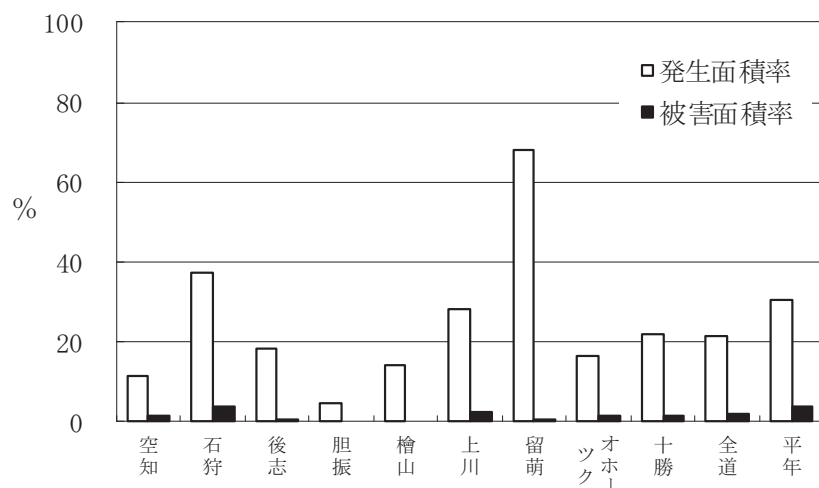
図2 小麦雪腐病の振興局別発生状況 (2023年4月)
