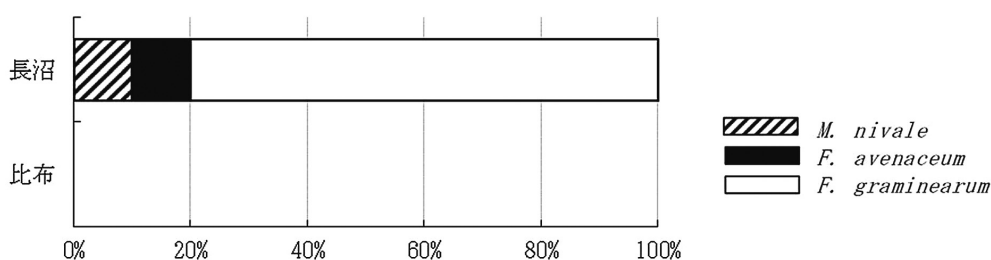
図8 予察ほにおける春まき小麦（「春よ恋」）の赤かび病菌種別割合（2023年）
