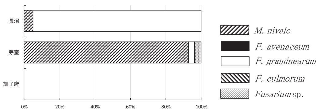
図6 予察ほにおける秋まき小麦の赤かび病菌種別割合（2023年）
