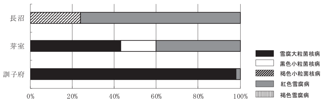
図 1 予察ほ（きたほなみ）における菌種別割合（2023年）
