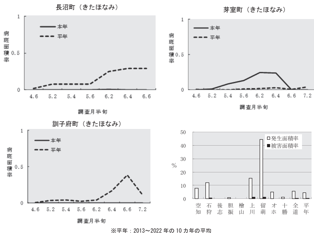
図5 予察ほおよび全道のうどんこ病発生状況（2023年）
