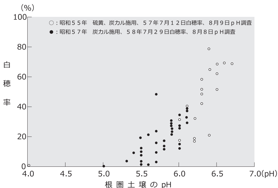
図23 根圏のpHと白穂の発病程度
