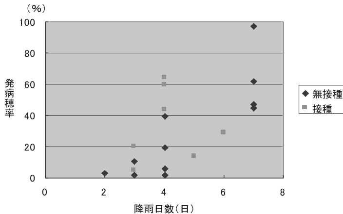
図16 開花始から15日間の降雨日数と発病率との関係 (1999~2006年、「ハルユタカ」、中央農試)
