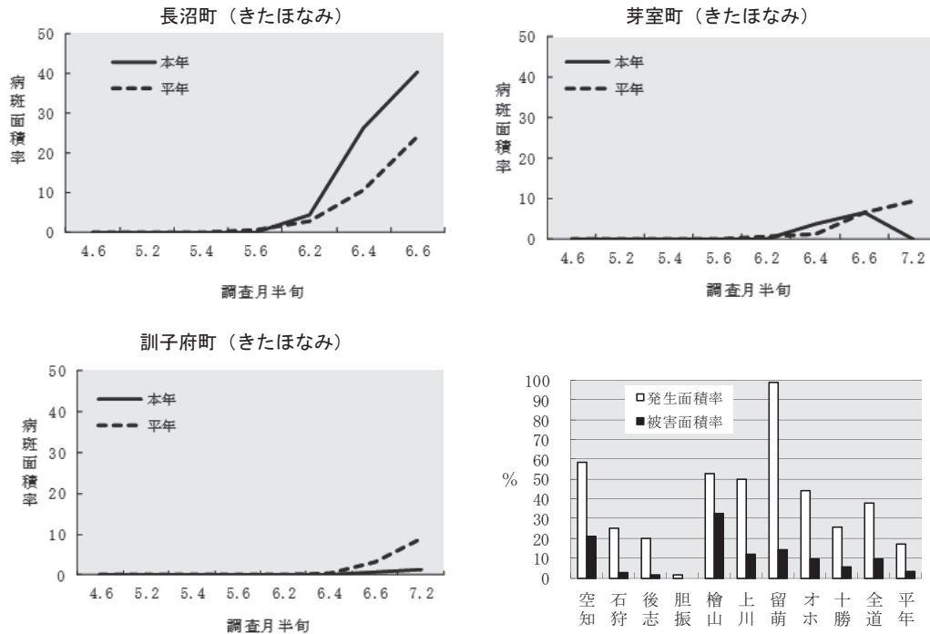
図4 予察ほおよび全道の赤さび病発生状況（2023年）
