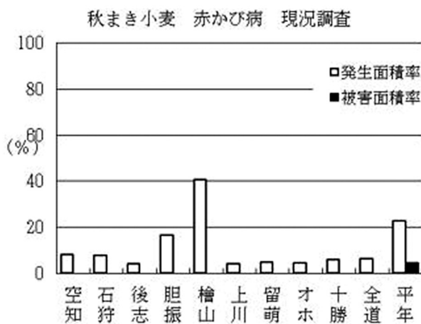
図7 振興局別の秋まき小麦赤かび病発生状況（2024年）
