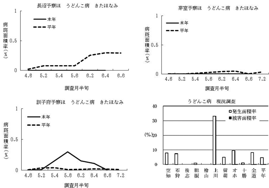
図5 予察ほおよび全道のうどんこ病発生状況（2024年）
