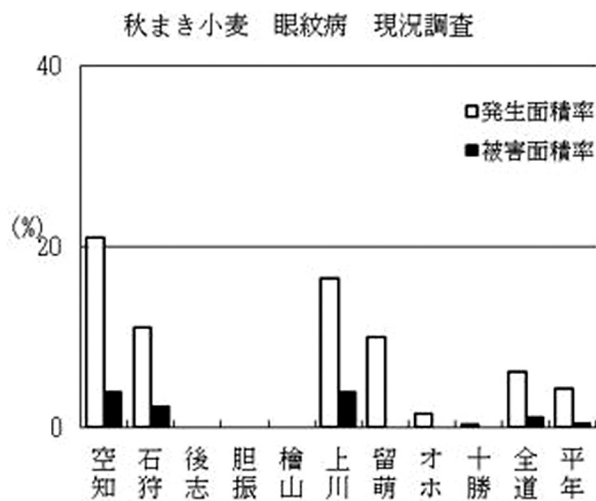
図10 振興局別の秋まき小麦眼紋病発生状況（2024年）
