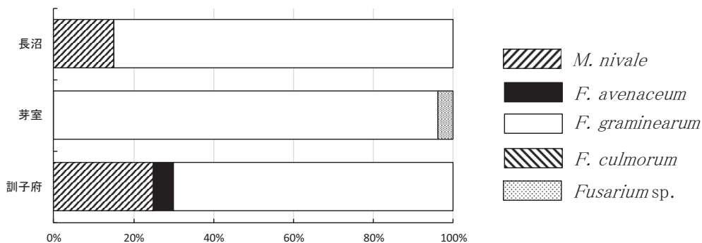
図6 予察ほにおける秋まき小麦の赤かび病菌種別割合（2024年）
