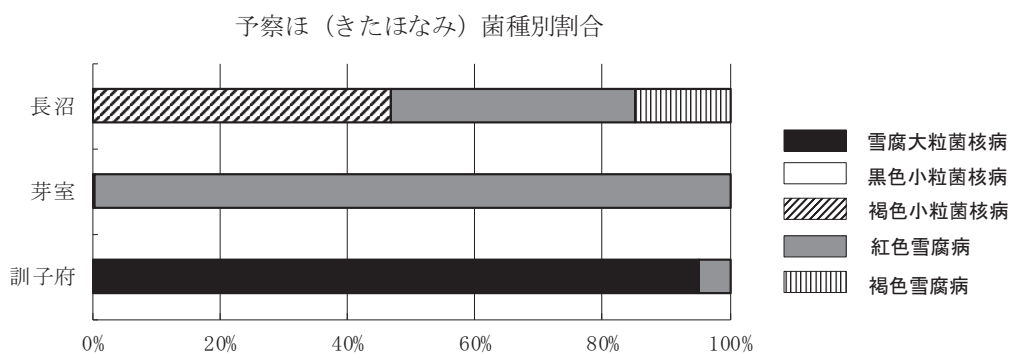
図1 予察ほ（きたほなみ）における菌種別割合（2024年）
