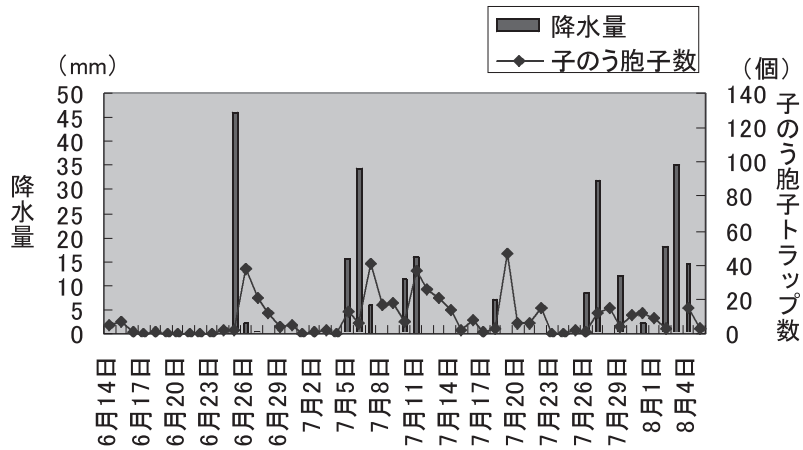
図20 子のう胞子トラップ数と降雨との関係 (2005年、春まき小麦)
