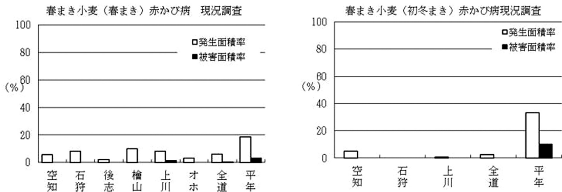
図9 振興局別の春まき小麦赤かび病発生状況（2024年、春まき・初冬まき）
