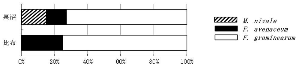
図8 予察ほにおける春まき小麦（「春よ恋」）の赤かび病菌種別割合（2024年）
